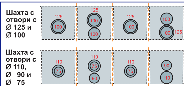
Ревизионна шахта за кабели
